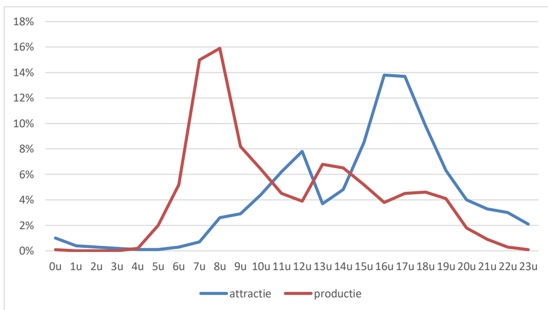
Figuur 5-6 Verdeling verplaatsingen over de dag
