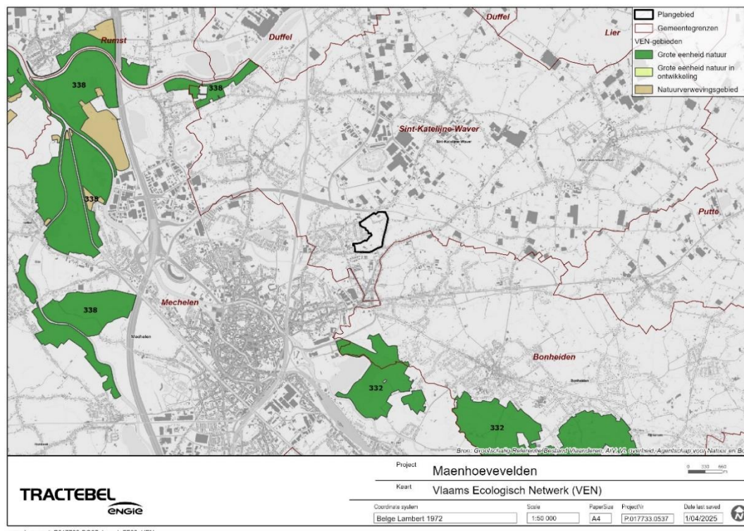
Figuur 5-54 VEN- en IVON-gebieden
