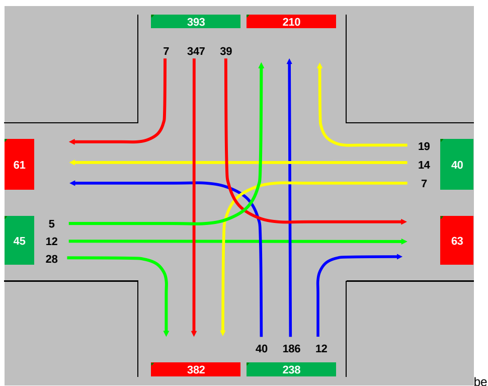
Figuur 5-16 Intensiteiten Berkelei X Meidoornstraat, referentie, ochtendspits (08:00-09:00)
