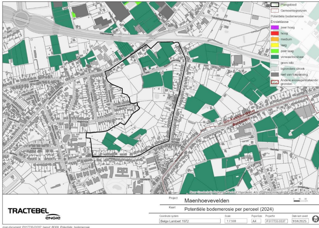
Figuur 5-47 Potentiële bodemerrosie per perceel (2024)
