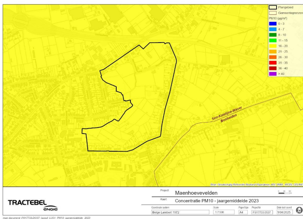
Figuur 5-37 Jaargemiddelde waarde voor de PM10-concentratie (bron VMM)
