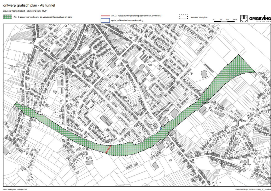
Figuur 4: grafisch plan deelplan A8-tunnel (bron: Provinciaal Ruimtelijk Uitvoeringsplan 'Afbakening Kleinstedelijk gebied Halle- cluster A8')
