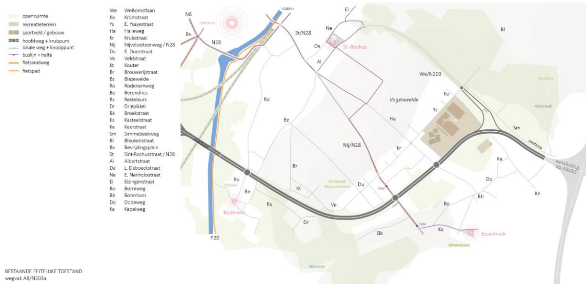
Figuur 25: Overzicht huidige feitelijke referentietoestand van de A8 in zijn omgeving ter vergelijking met de inrichtingsalternatieven.
