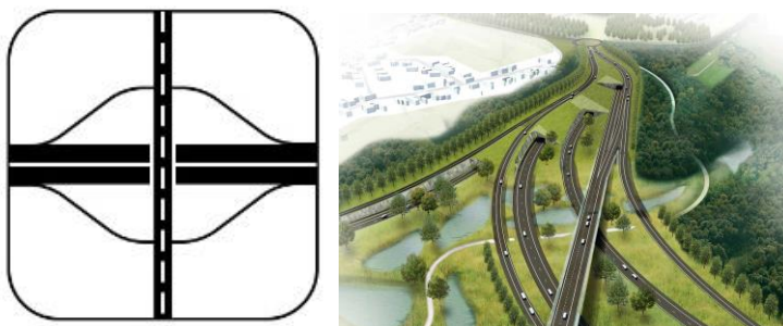
Figuur 14: Configuratie van een compact 'Hollands Complex' versus de geplande 'spaghettiknoop' volgens het PRUP KSG Halle.
