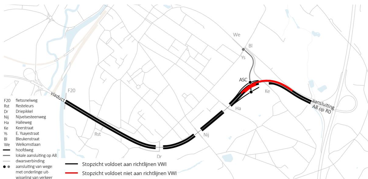
Figuur 50: Visuele weergave van de analyse voor stopzicht in alternatief 1 mits toepassing milderende maatregel
