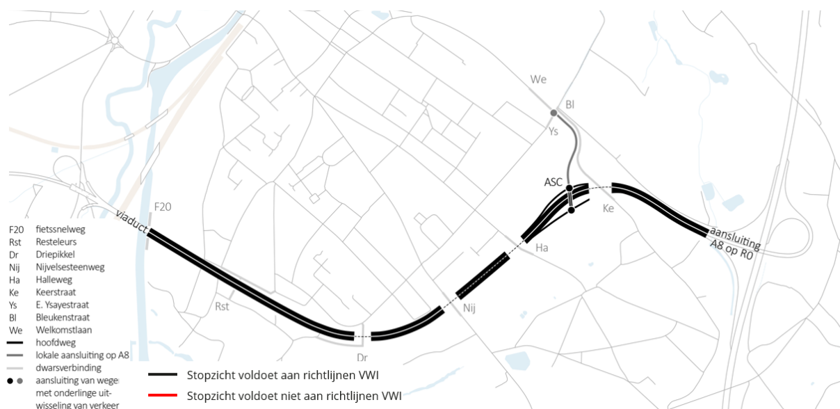
Figuur 51: Visuele weergave van de analyse voor stopzicht in alternatief 1 (ontwerpsnelheid 70km/u)
