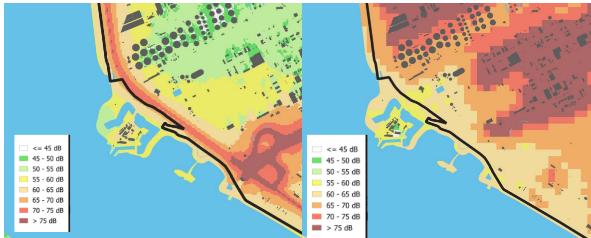
Figuur 4-26: Geluidsbelastingsskaarten Lden agglomeratie Antwerpen en de haven Antwerpen (2023) wegverkeer (links) en industrie (rechts)
