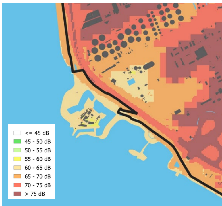
Figuur 4-27: Algemene (Weg + Spoor + Industrie) Lden geluidsbelastingsskaarten (2023)
