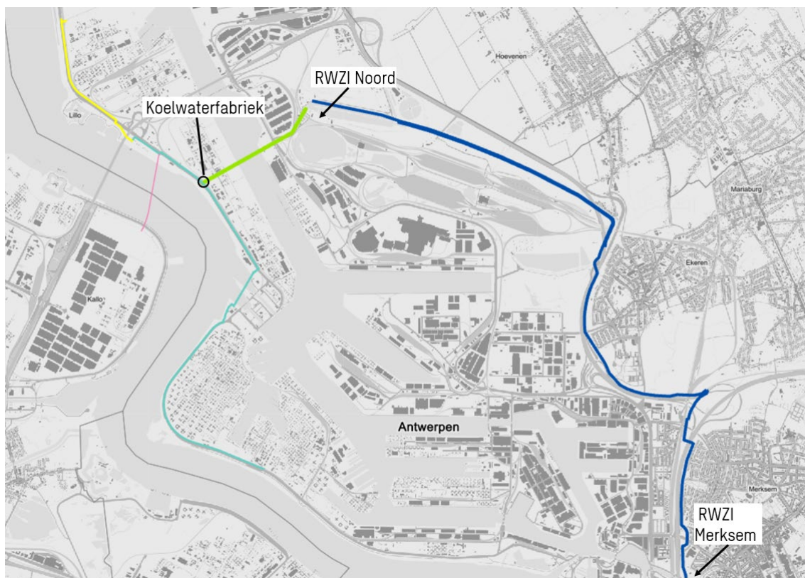
Figuur 4-3: Indicatieve ligging van het koelwaternetwerk in de Antwerpse haven (in ontwerp)
